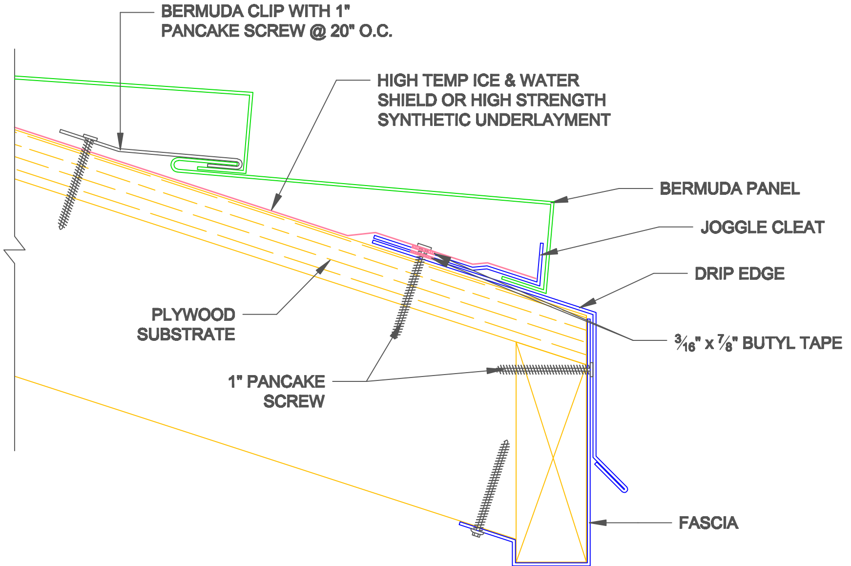
BERMUDA DRIP EDGE W/ JOGGLE
